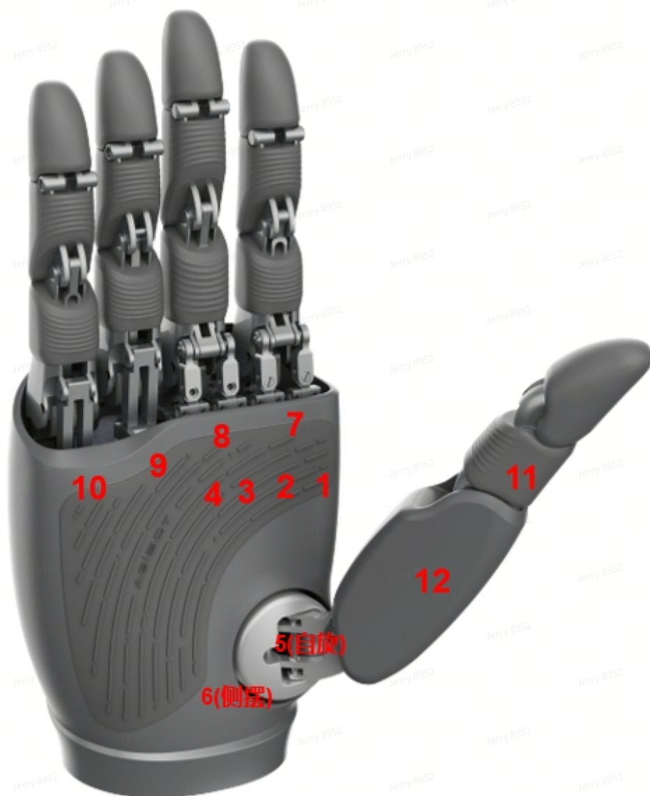
专业款灵巧手 主动自由度示意图
